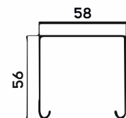
BÄRPROFIL
