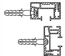
DIREKTMONTERING
