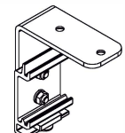
VÄGGKONSOL AV TYPEN "F"
